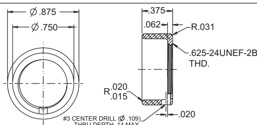
OTTO P/N C300793
