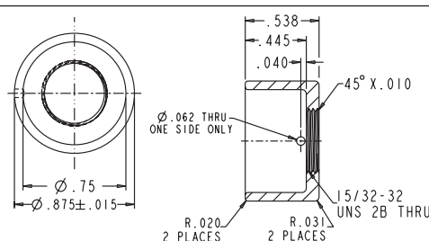
OTTO P/N C300428
