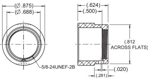
OTTO P/N C300871
